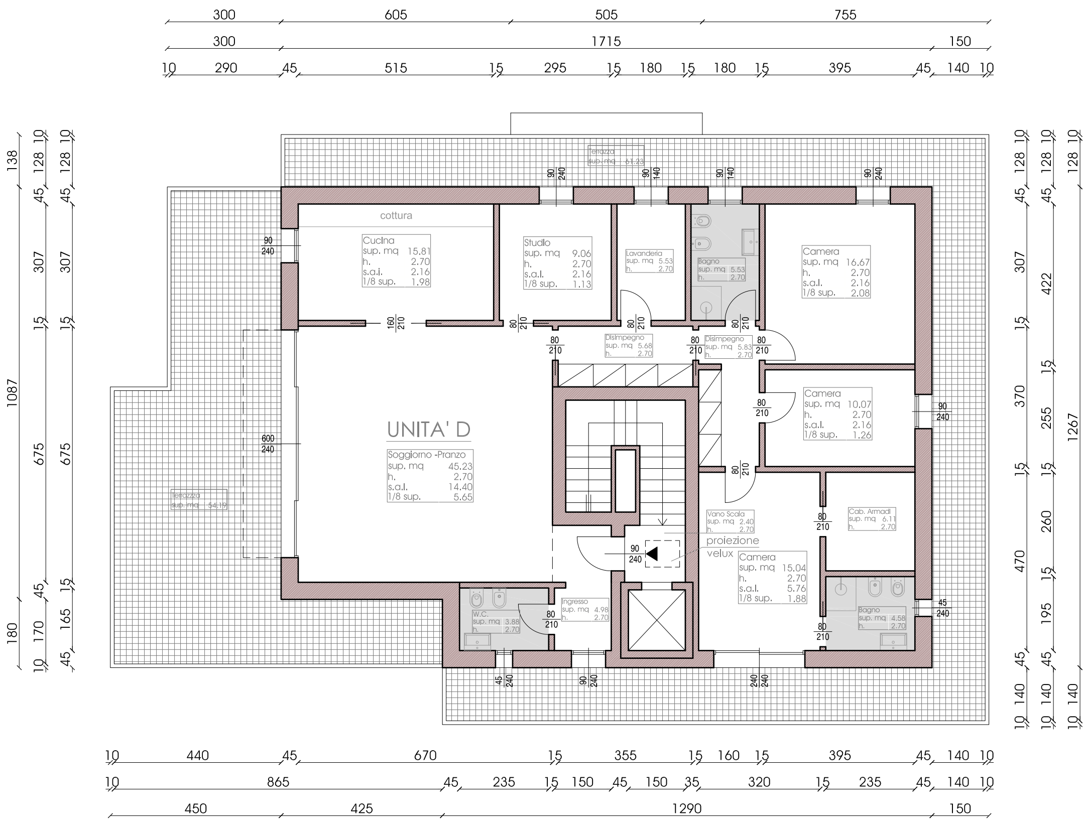
PIANTA PIANO SECONDO 1.100
