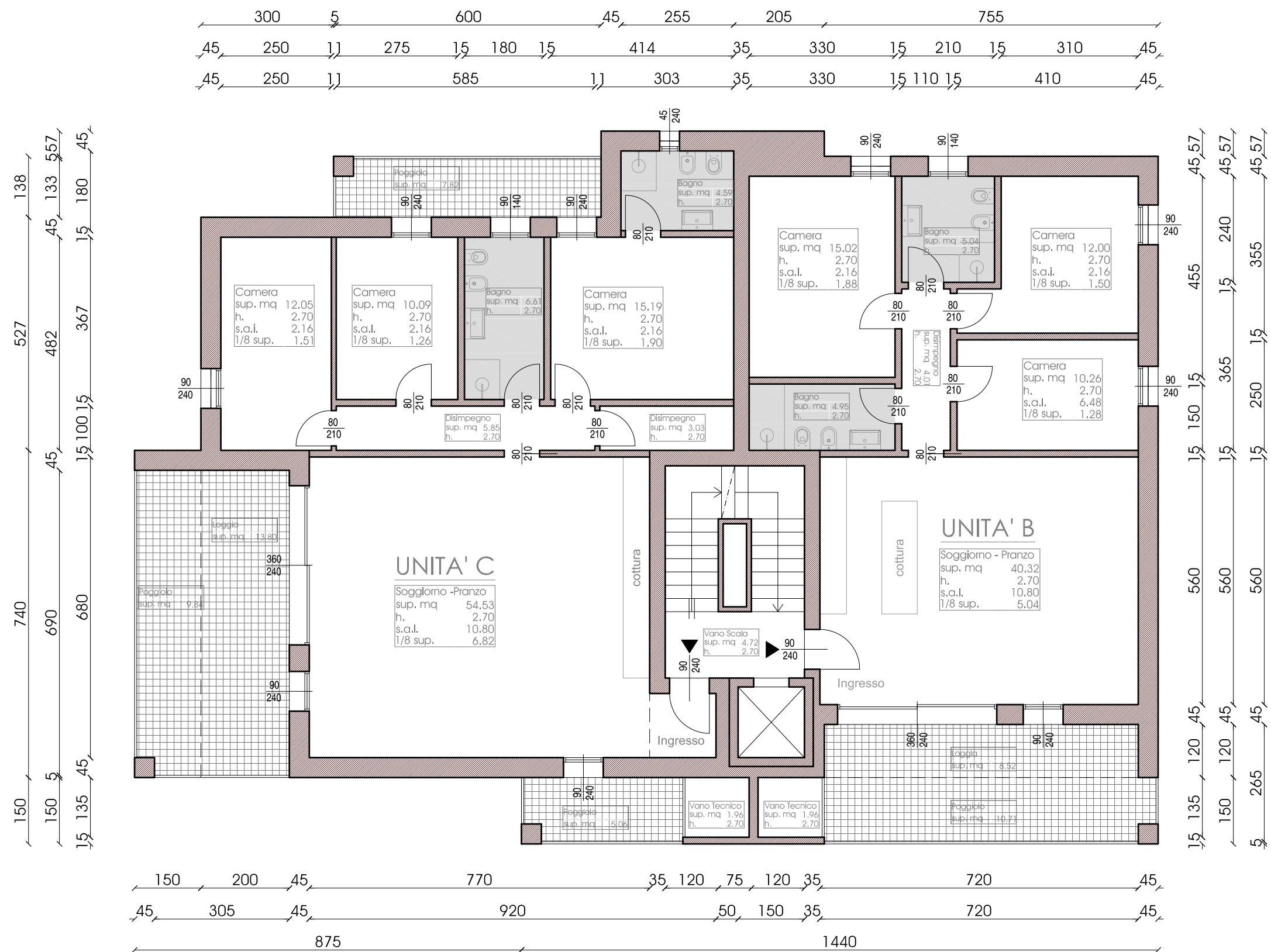
PIANTA PIANO PRIMO 1.100
